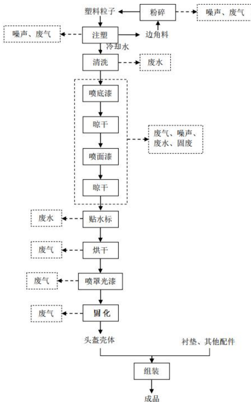
图 3.5-1 生产工艺流程图
