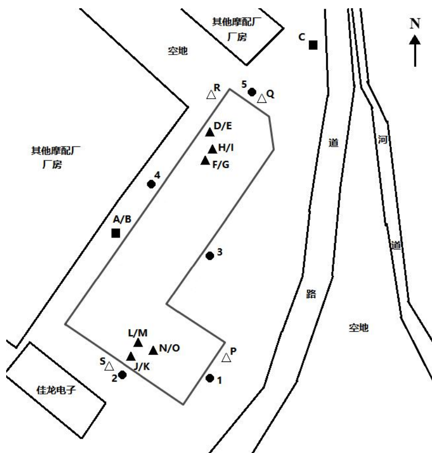
图 5.1-1 项目竣工环境保护验收监测点位图
