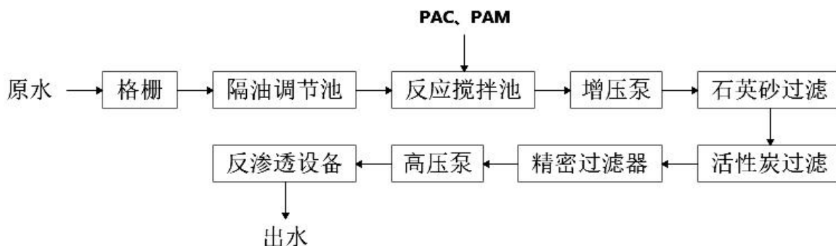
图 4.2-1 废水处理工艺流程图
