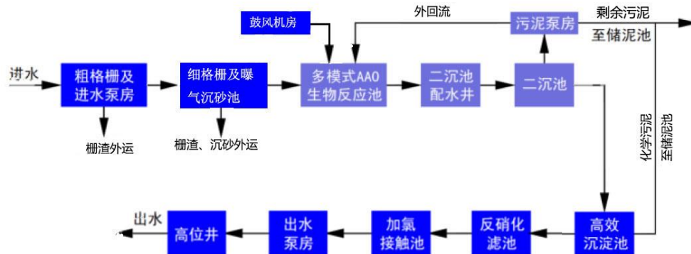
图 4-12 江南污水处理厂扩容提标工程工艺流程图（在建）
