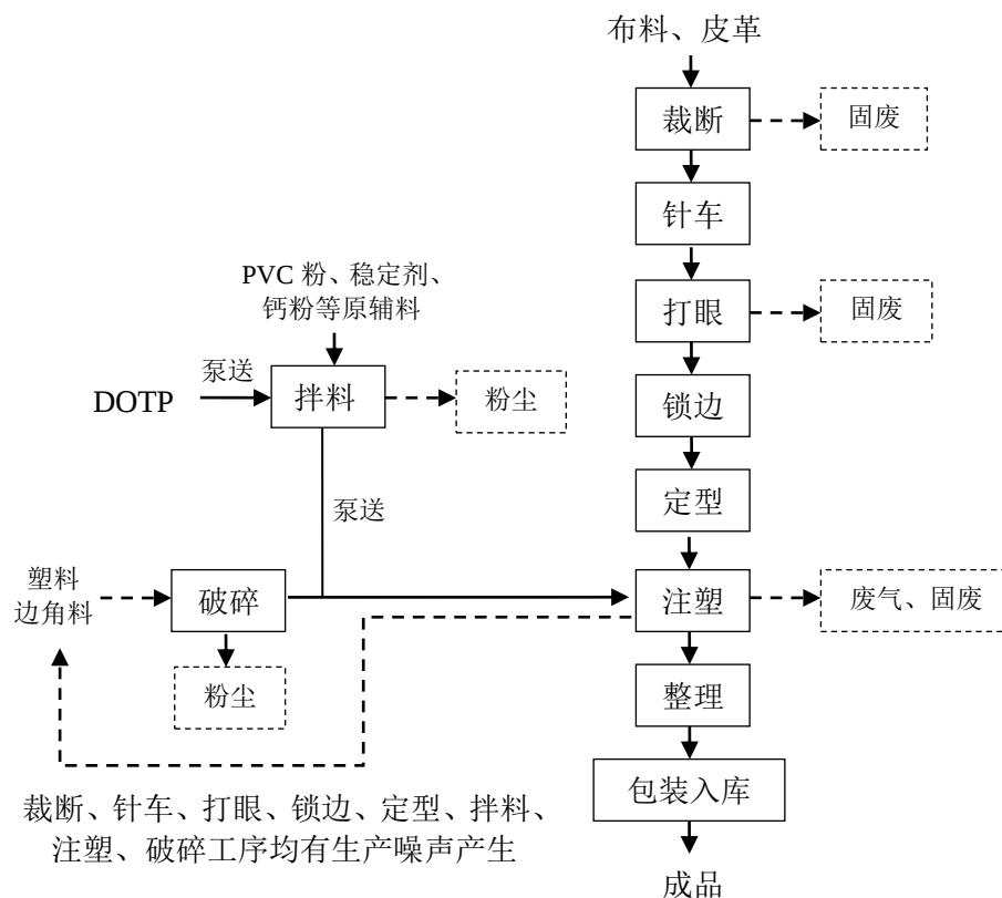
图 2-2 注塑工艺流程图
