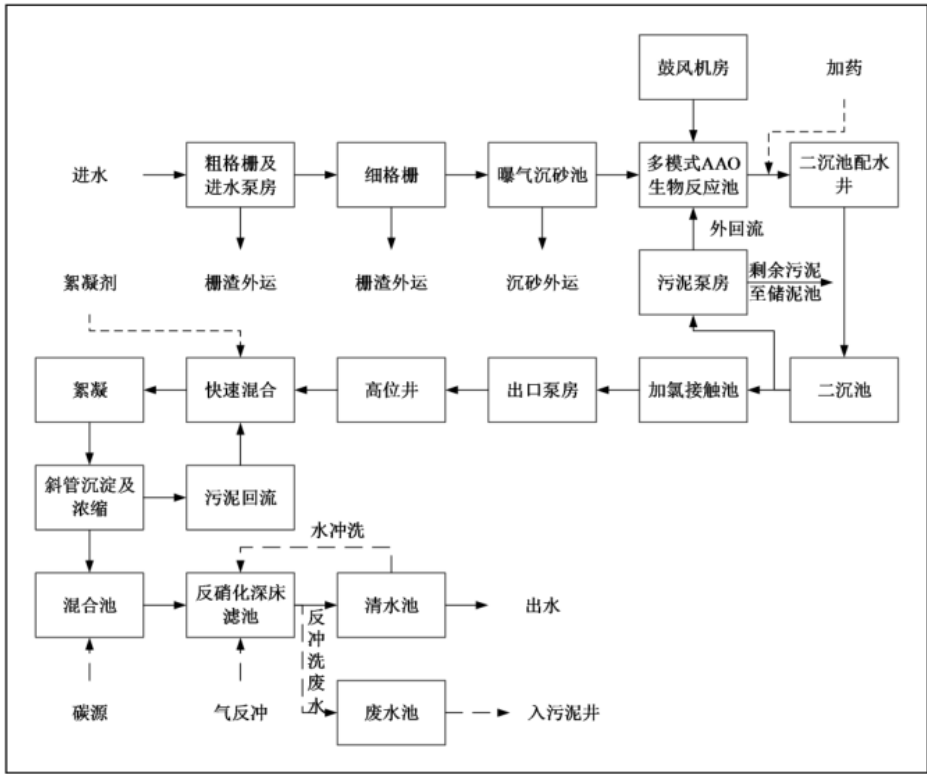
图 4-11 江南污水处理厂一期工程工艺流程图
