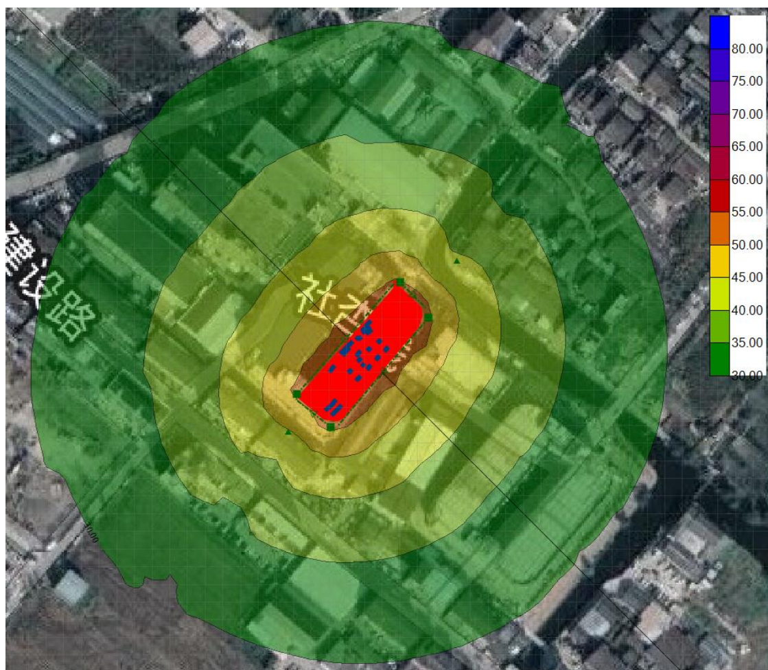
图 4-5 昼间噪声预测结果图
