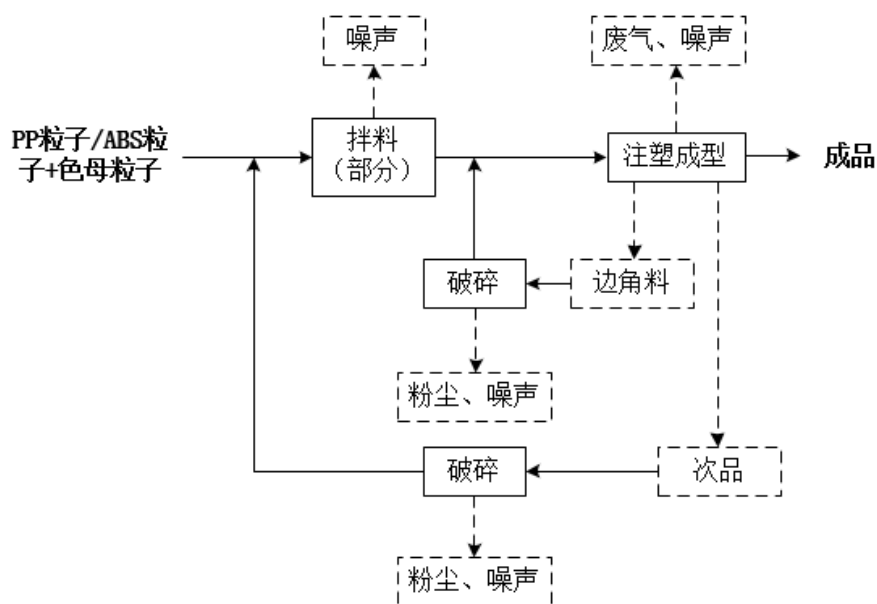
图 2-3 塑料日用品生产工艺流程图
