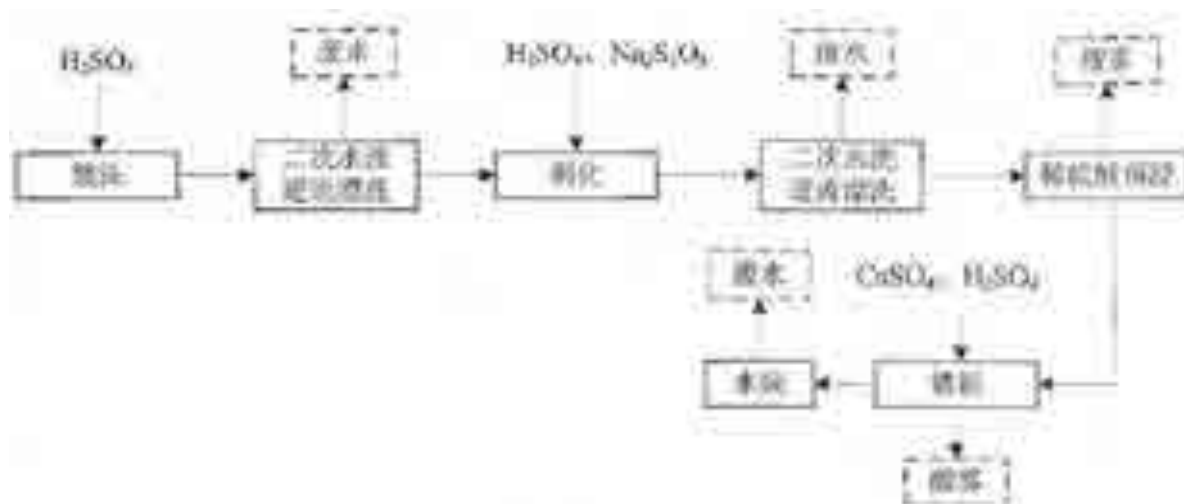
图 3.2-5 图形电镀工艺流程及产污环节图
