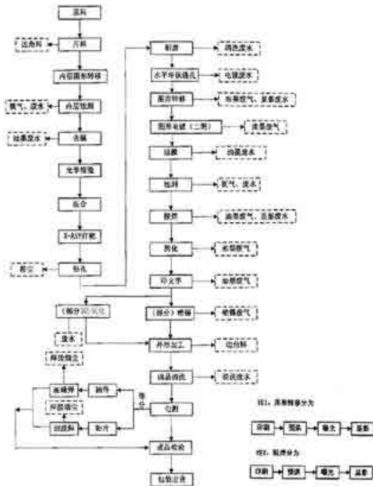
图 3.2-3 高密度多层板生产工艺流程及产污环节图
