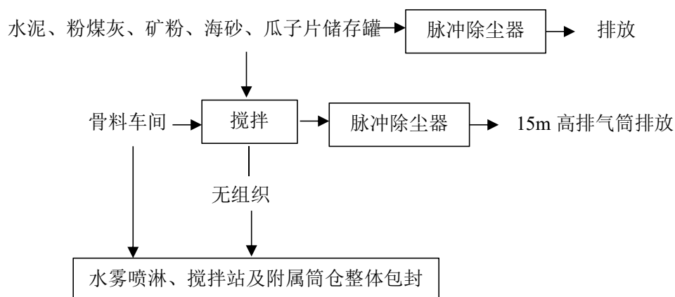
图 4-1 项目废气治理措施示意图
