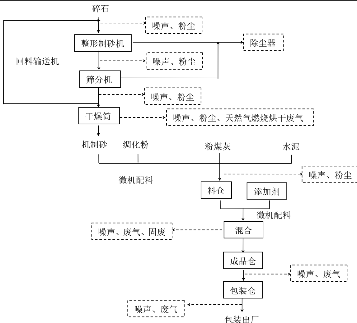
图 2-1 干式制砂+干混砂浆一体机生产线工艺流程图
