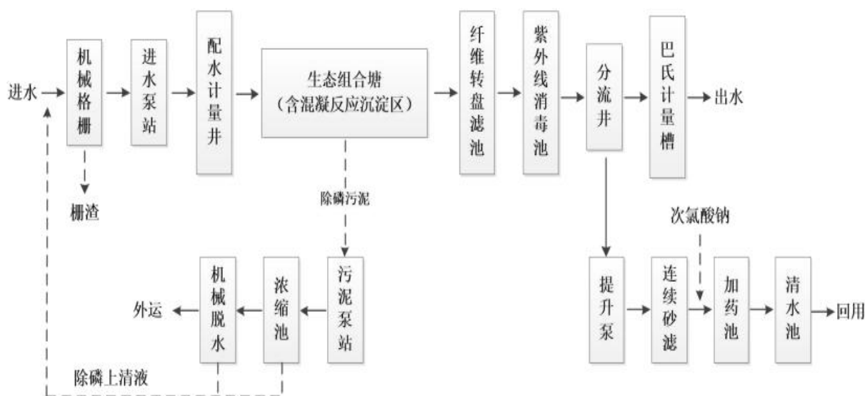
图 4-2 污水处理工艺流程
