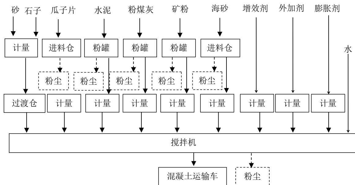
图 2-2 混凝土生产工艺
