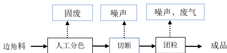
图 2-2 项目主要工艺流程图
