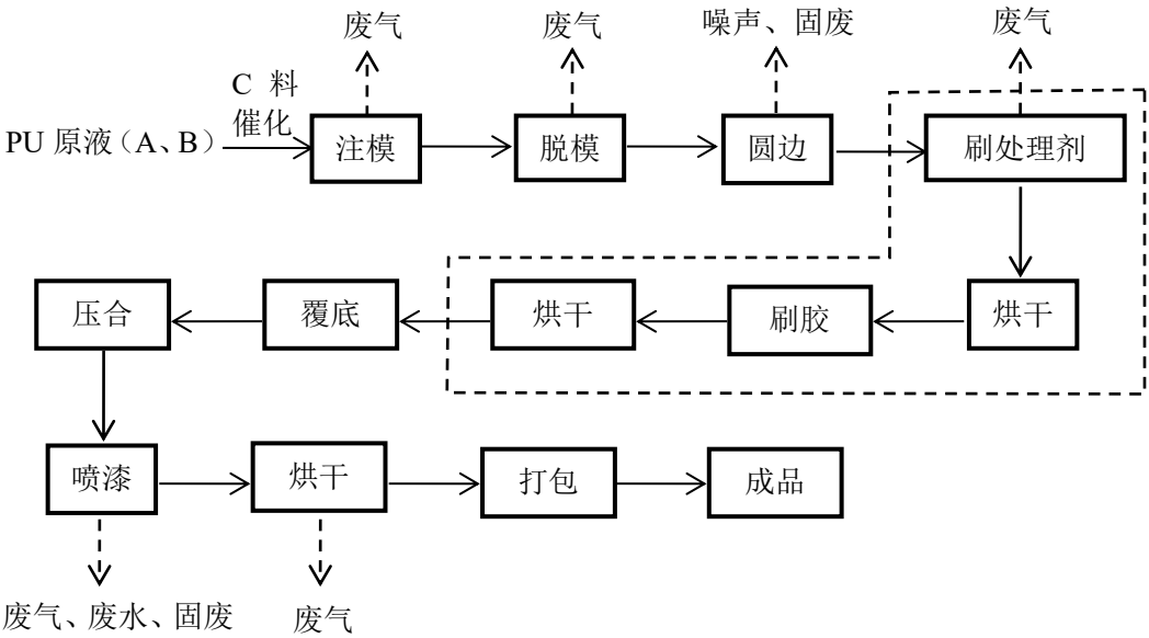
图 2-3 PU 鞋底生产工艺流程及产污环节
