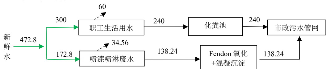
图 2-1 项目建成后全厂水平衡图 (t/a)
