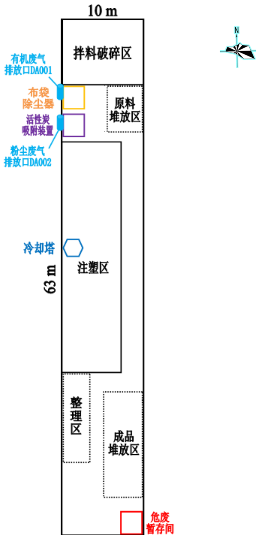
附图 9 嘉菲鞋厂平面布置图
