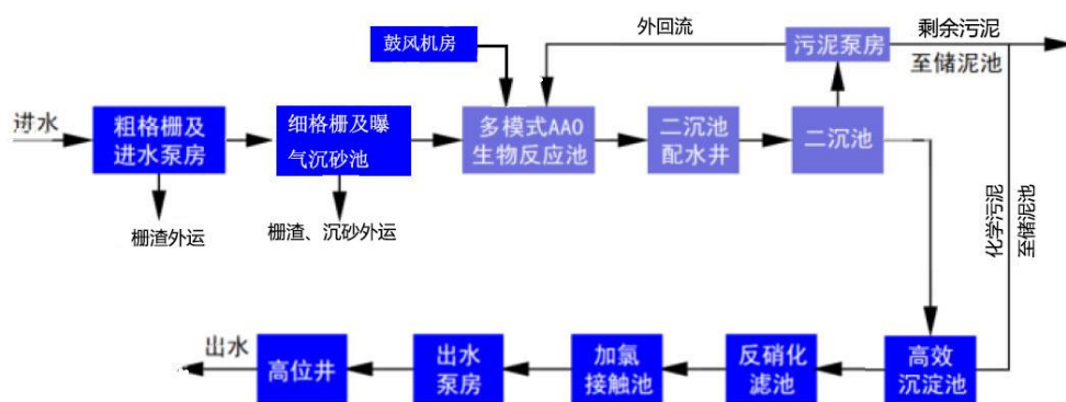
图 4-1 江南污水处理厂污水处理工艺流程图
