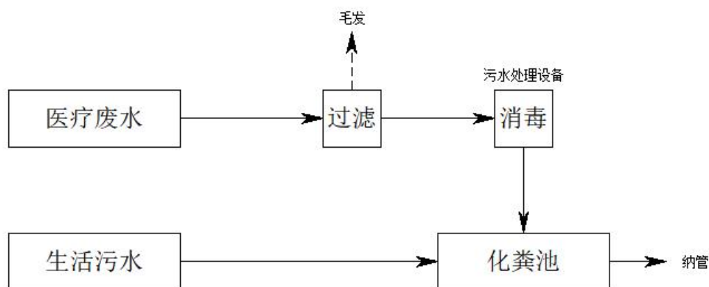
图 4-1 废水工艺流程图
