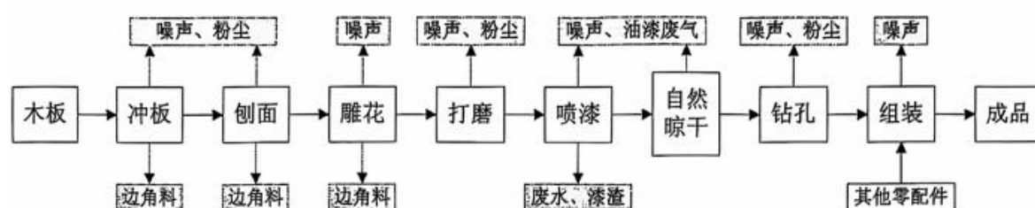
图 2-3 卫浴洁具（橱柜等）、浴柜原审批生产工艺流程图（目前停产中）
