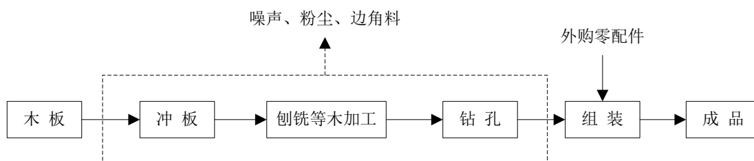
图 2-7 卫浴洁具（橱柜等）、浴柜生产工艺流程图
