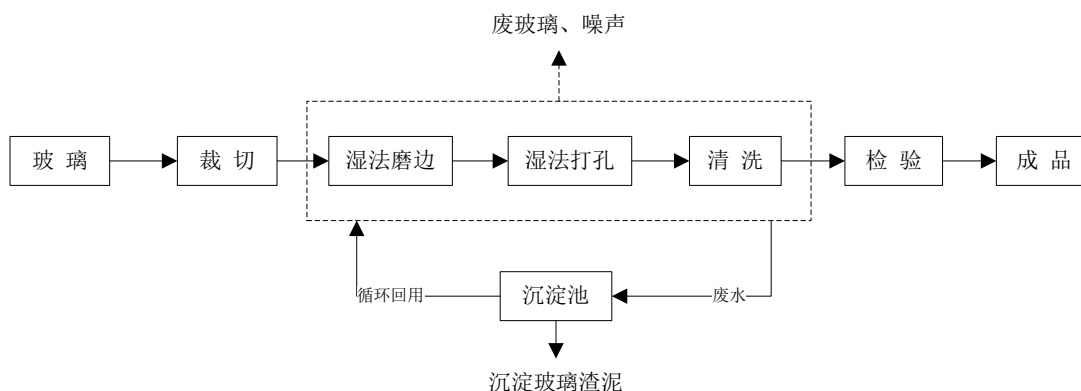
图 2-8 美容镜生产工艺流程图
