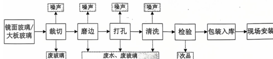
图 2-4 美容镜、淋浴房原审批生产工艺流程图
