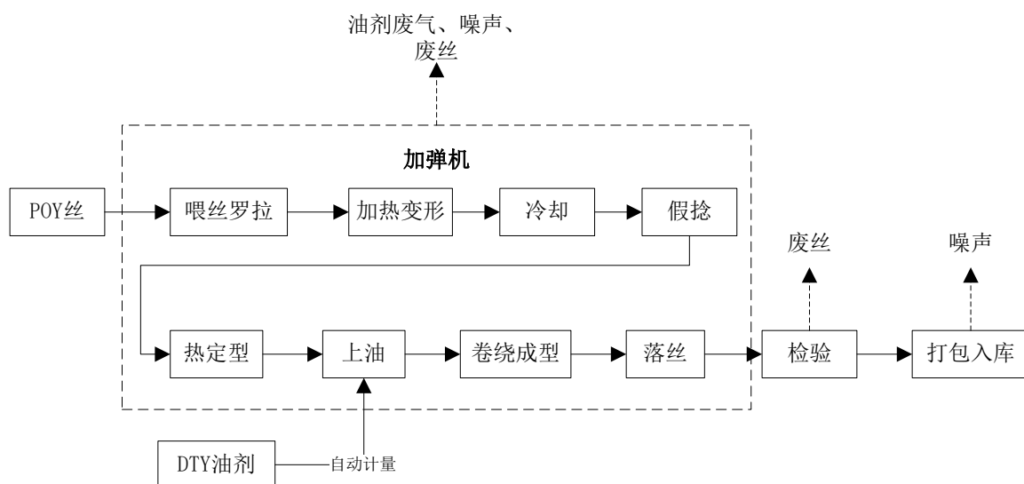
图 2-2 高档加弹丝生产工艺和产污点流程图
