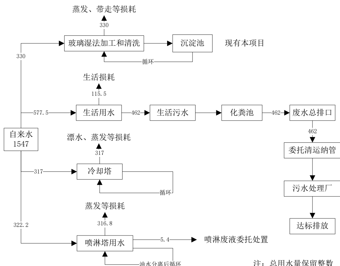
图 2-1 改建后厂区水平衡分析图 (单位: t/a)
