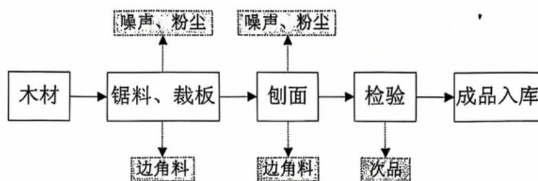
图 2-6 木门原审批生产工艺流程图（实际未投产）
