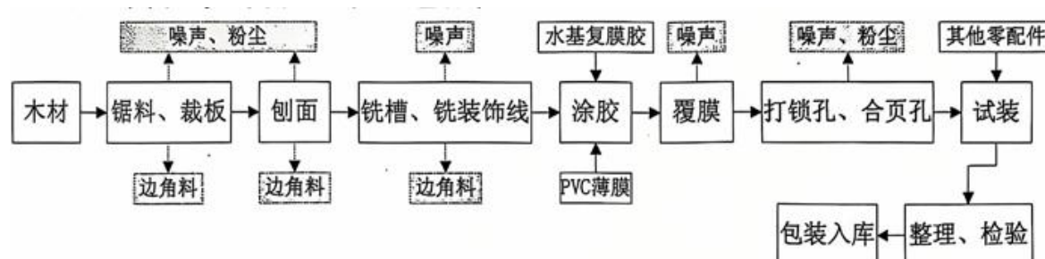
图 2-5 木门原审批生产工艺流程图（实际未投产）
