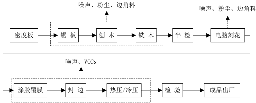
图 2-7 免漆木质家具和免漆木门原审批生产工艺流程图(未曾投产)
