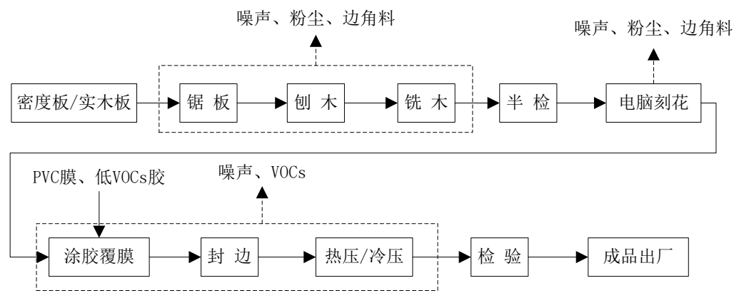
图 2-3 免漆装饰门和免漆板材生产工艺流程图
