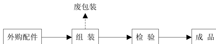
图 2-12 卫浴五金组装原审批生产工艺流程图（未曾投产）
