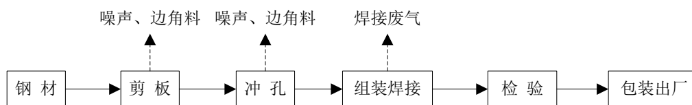
图 2-14 结构性金属制品原审批生产工艺流程图（未曾投产）
