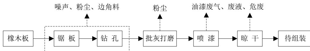
图 2-10 浴柜原审批生产工艺流程图（未曾投产）
