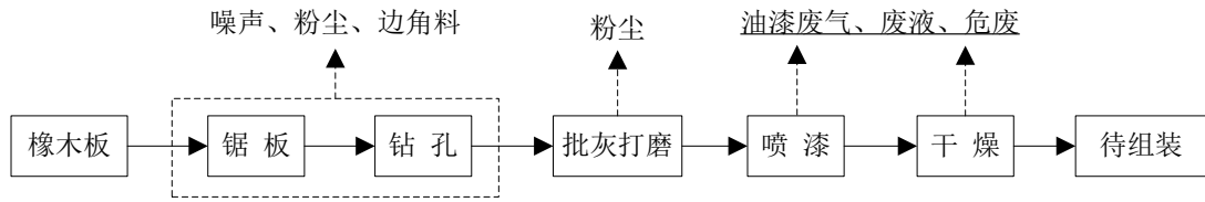
图 2-5(1) 浴柜原审批生产工艺流程图
