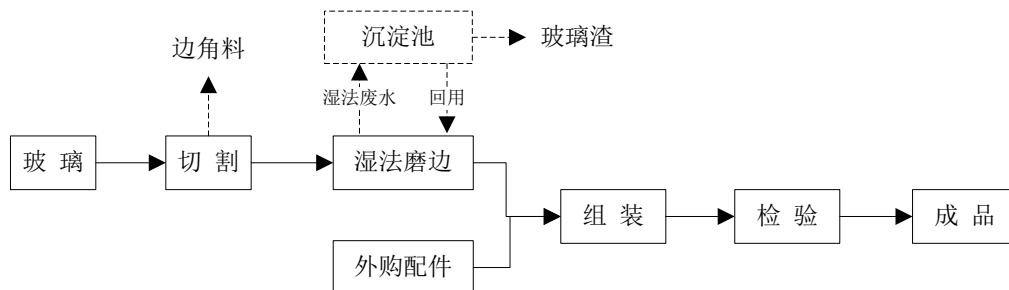
图 2-11 淋浴房组装原审批生产工艺流程图（未曾投产）
