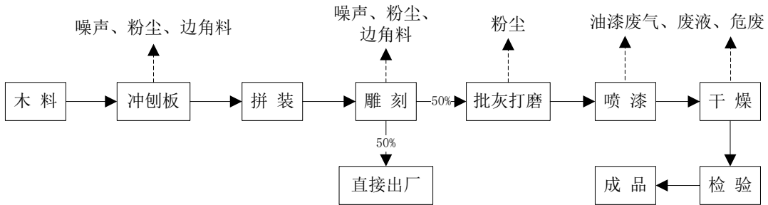
图 2-9 实木门原审批生产工艺流程图(未曾投产)
