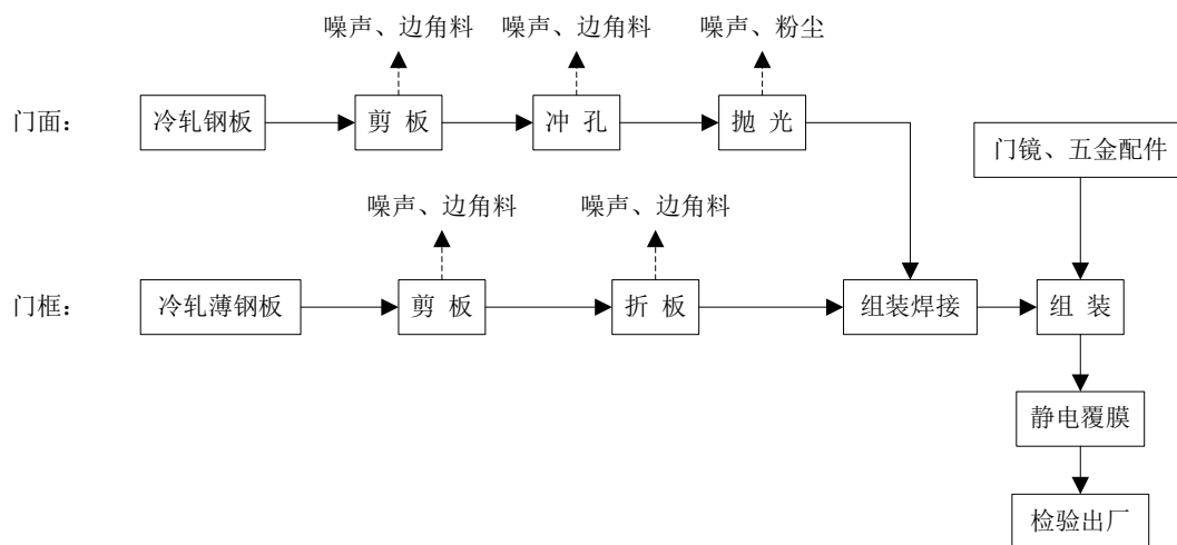
图 2-13 防盗门原审批生产工艺流程图（未曾投产）
