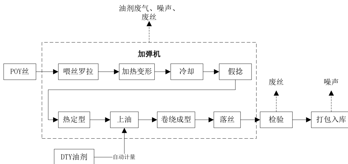
图 2-2 功能性环保纤维假捻变形生产工艺和产污点流程图
