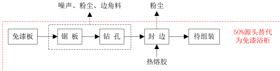
图 2-5(2) 源头替代后浴柜（免漆类）生产工艺流程图
