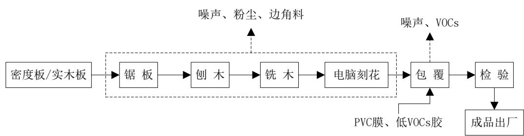
图 2-4 免漆木线条生产工艺流程图
