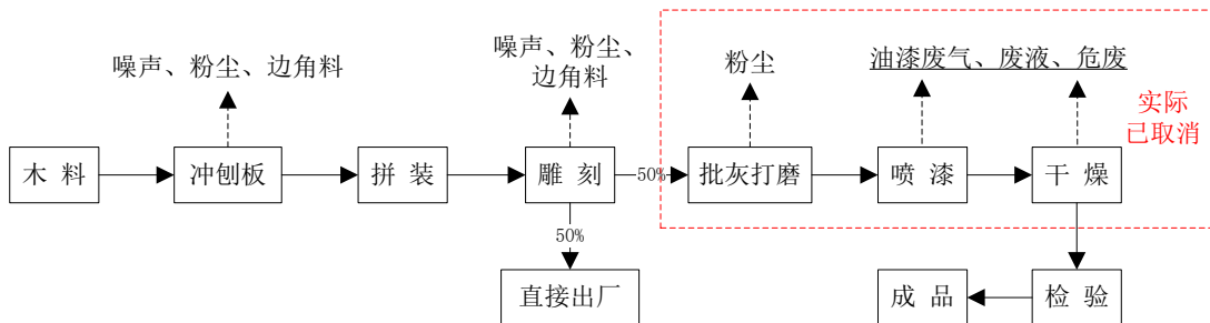
图 2-6 实木门生产工艺流程图
