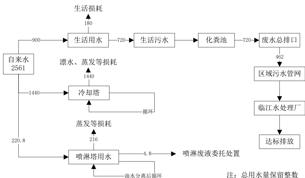
图 2-1 本项目厂区水平衡分析图 (单位: t/a)
