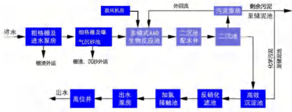
图 4-1 瑞安市江南污水处理厂工艺流程图
