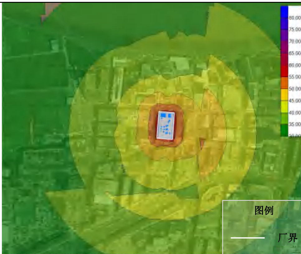
图 4-3 昼间噪声预测结果图
